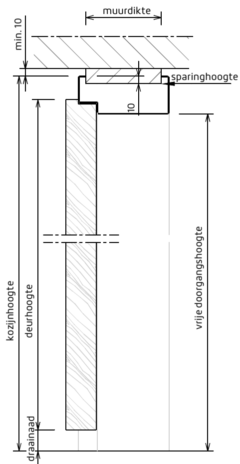
Verticale doorsnede
